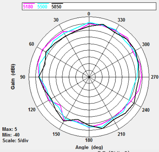
5G (PHI=0)
