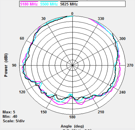
5G (PHI=90)
