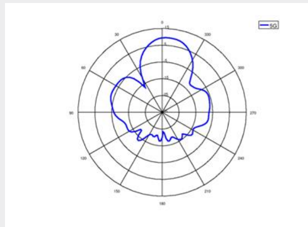
5G (PHI=90)
