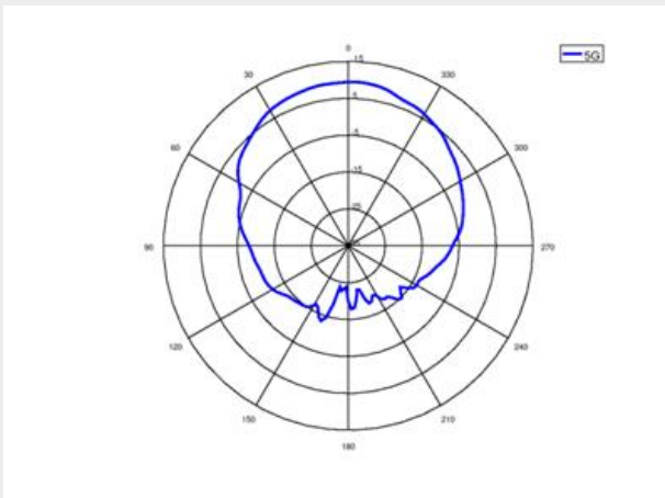
5G (PHI=0)
